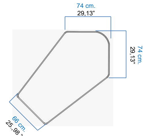
BANQUETTE D'ANGLE PROF.98 CORNER ARMLESS SOFA DEPTH.98 BANQUETA DE ÁNGULO PROF.98
